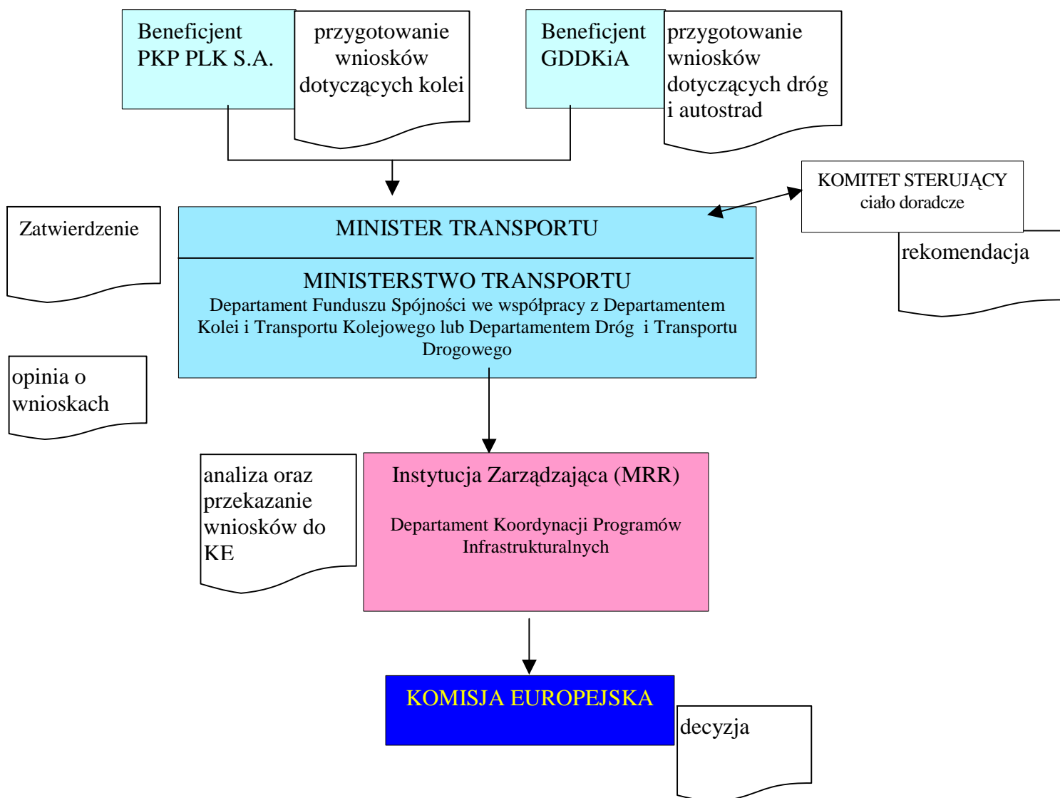
RYS 3. SCHEMAT PROCESU WYBORU, OCENY I PRZYGOTOWANIA PROJEKTÓW FUNDUSZU SPÓJNOŚCI W SEKTORZE TRANSPORTU
